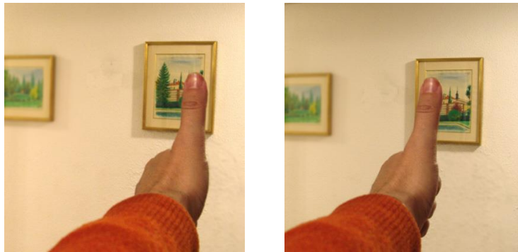
Fig. 1a: Con el brazo extendido miramos la posición del pulgar respecto al fondo, primero con el ojo izquierdo (cerrando el derecho) y después al revés, Fig. 1b: lo miramos con el ojo derecho (con el izquierdo cerrado).
