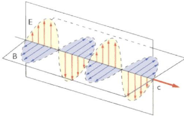
Fig. 2: Luz polarizada
