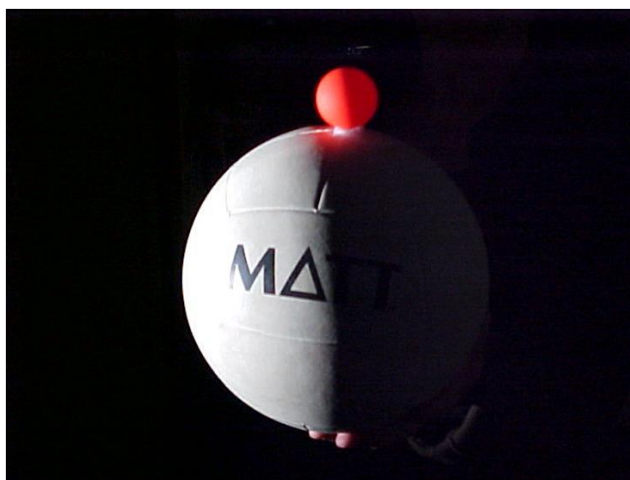
Fig. 5: Un foco ilumina dos esfera de la misma forma y produce las mismas zonas de luz y sombra
