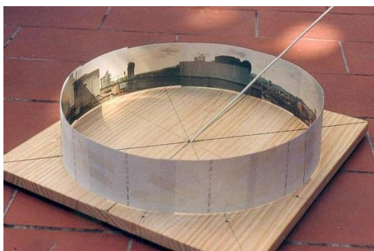
Fig. 13: Con el eje del mundo
