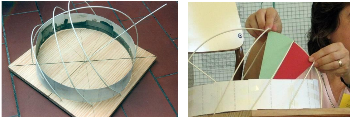
Fig. 19: Trayectorias del Sol el primer día de cada estación. Los puntos de salida y puesto no coinciden salvo dos días: el día de los equinoccios. Fig. 20: El ángulo entre dos trayectorias del primer día de dos estaciones consecutivas es de 23.5^\circ
