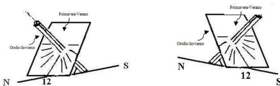
Fig. 23: Reloj ecuatorial en estación (hemisferio norte). Fig. 24: Reloj ecuatorial en estación (hemisferio sur).
