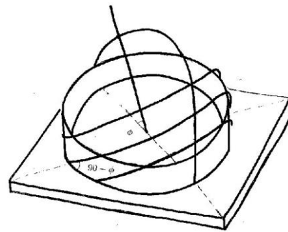
Fig. 12: Modelo mostrando con la latitud y la colatitud
