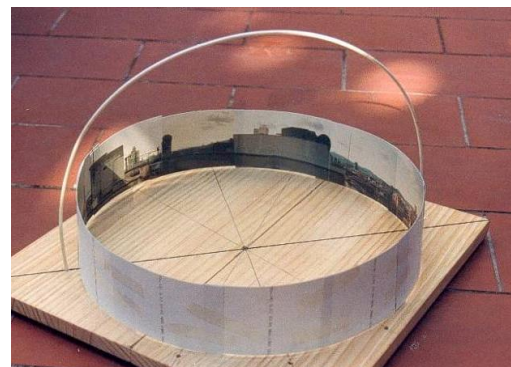
Fig. 14: Con el meridiano del lugar
