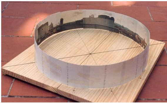
Fig. 11: El horizonte local
