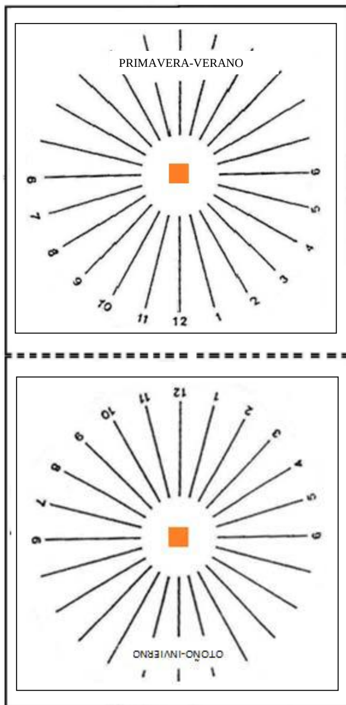
Fig. 25: Recortable del reloj ecuatorial
