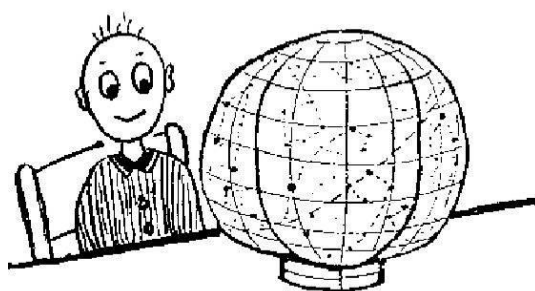
Fig. 9: La esfera celeste desde el exterior.
