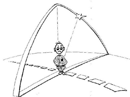
Fig. 10: La esfera celeste desde el interior
