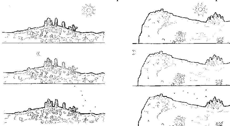
Fig. 27a: Horizonte Noroeste de Barcelona.
